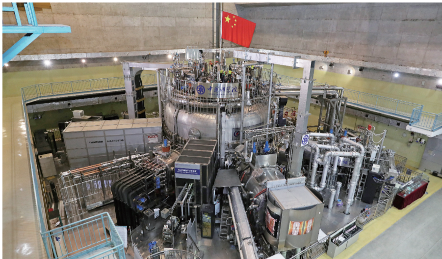
全超导托卡马克核聚变实验装置(EAST)
