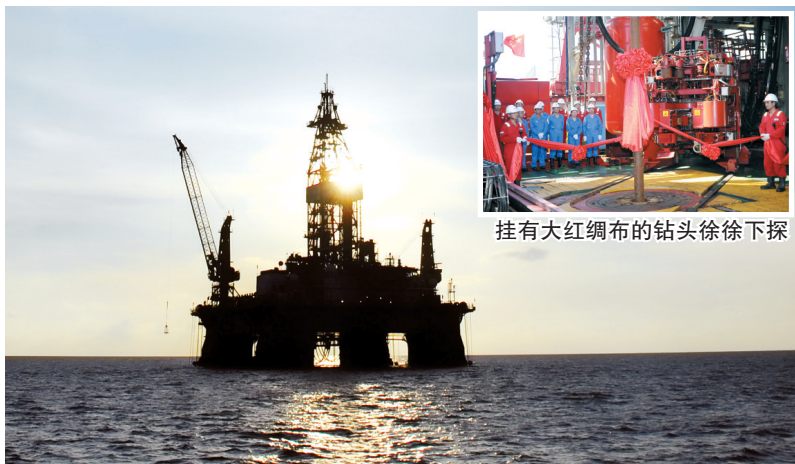
在海面上的“海洋石油981”深水钻井平台
