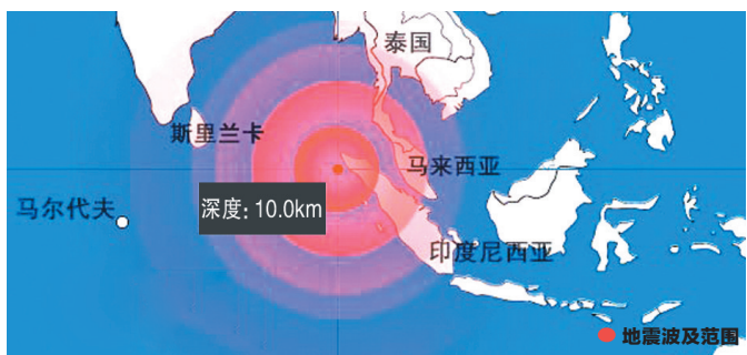
印尼8.5级地震示意图
