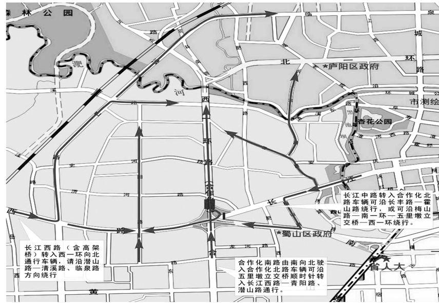
合作化北路淠河路口封闭施工期间交通组织示意图
