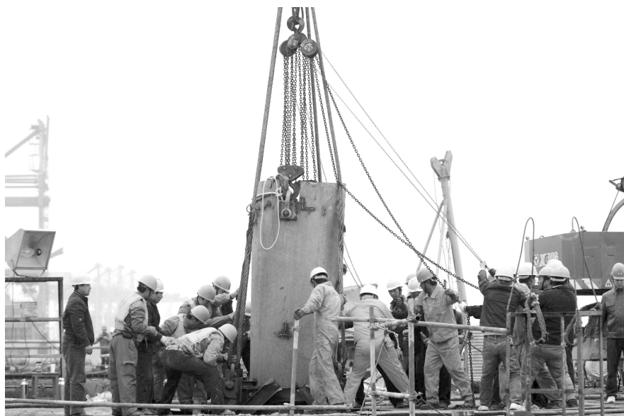
钢护筒被吊起
